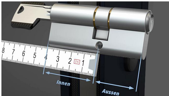
Zylinderlängenbestimmung im ausgebauten Zustand
